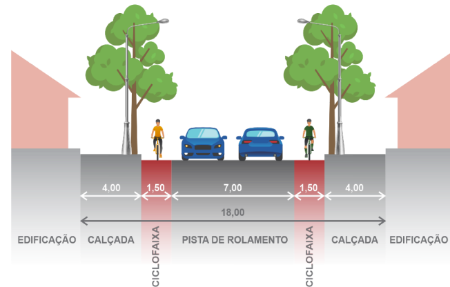
Via Arterial Tipo 2
