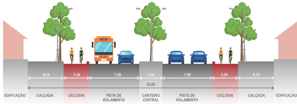
Via Arterial Tipo 2
