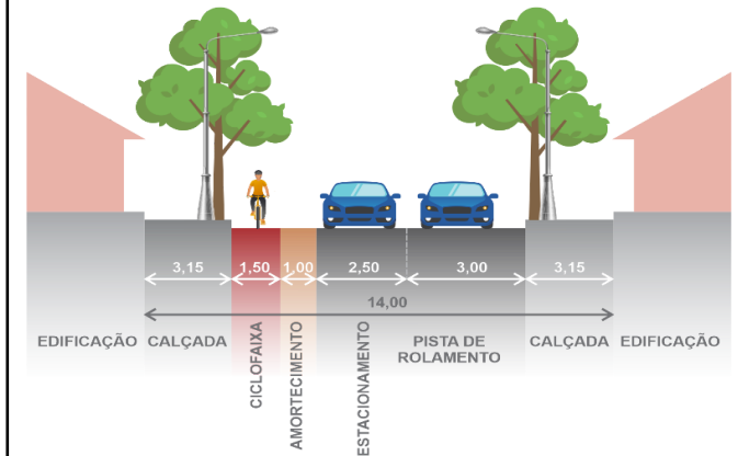
Via Coletora Tipo 2
