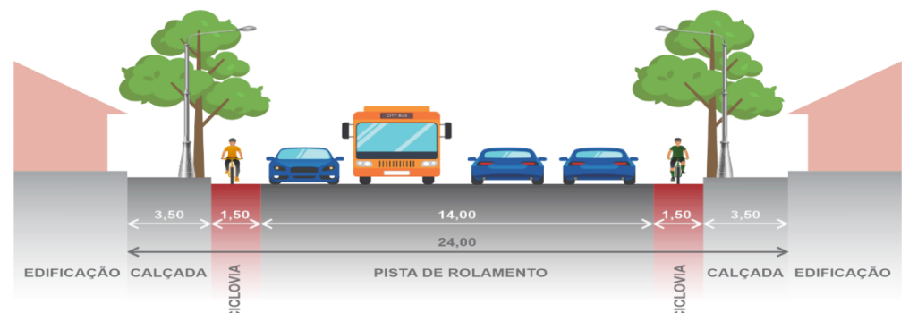
Via Coletora Tipo 1
